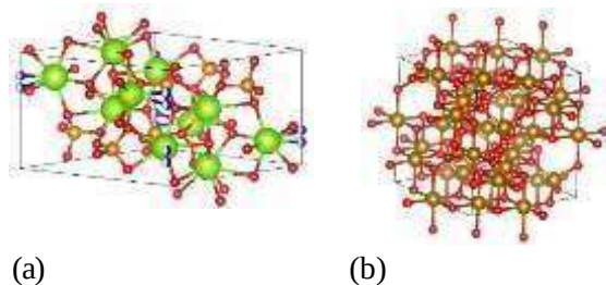
Gambar 7 Struktur kristal (a) HAp, dan (b) \text{Fe}_3\text{O}_4
