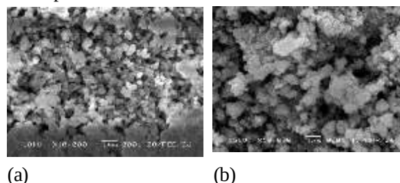
Gambar 8 Hasil karakterisasi SEM (a) HAp, (b) Komposit HAp/ \text{Fe}_3\text{O}_4 pada perbesaran 10.000\times
