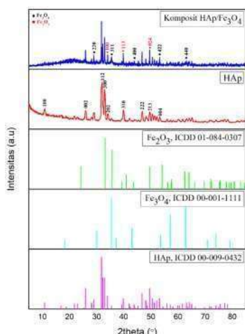
Gambar 6 Pola XRD dari HAp dan Komposit HAp/Fe 3 O 4
