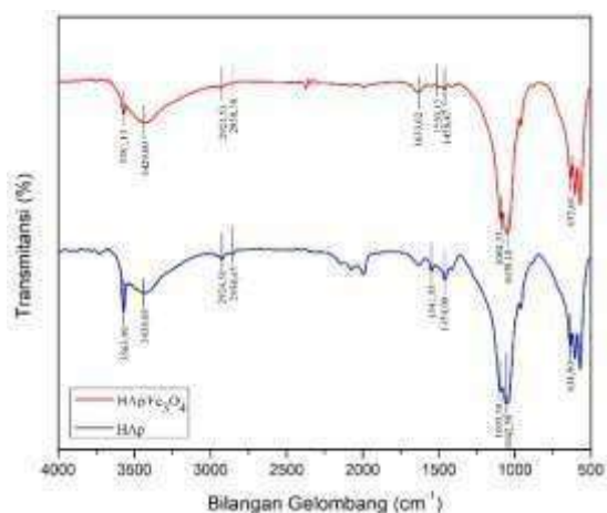
Gambar 5 Spektrum FTIR hidroksiapatit dan komposit HAp/ \text{Fe}_3\text{O}_4
